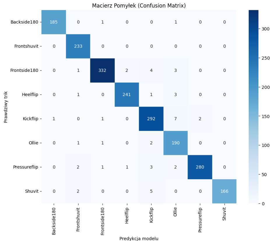
Rysunek 5.2. Macierz pomyłek klasyfikatora na zbiorze testowym, Źródło: [opracowanie własne].
