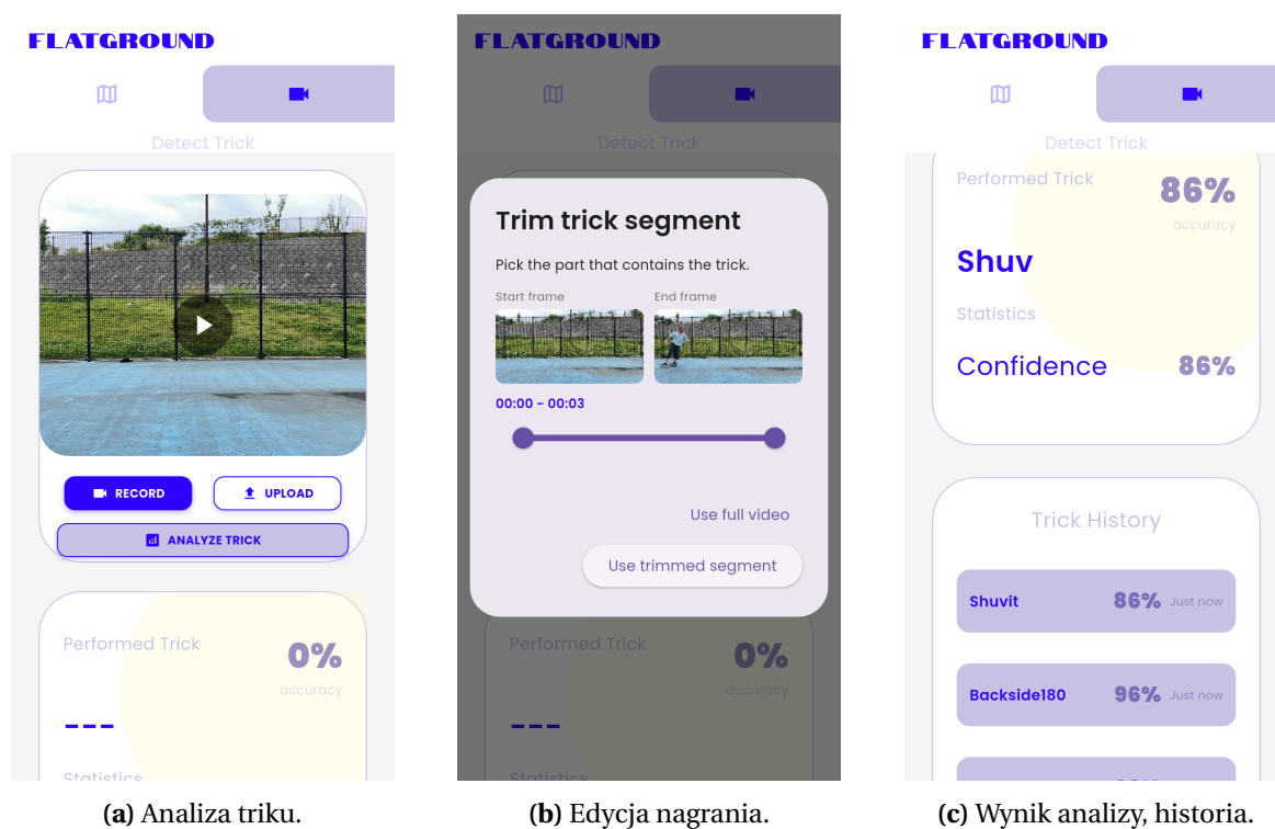
Rysunek 6.3. Ekrany zakładki analizy trików deskorolkowych, Źródło: [Opracowanie własne].
